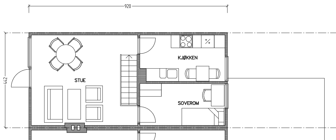
Plan 1. etasje
